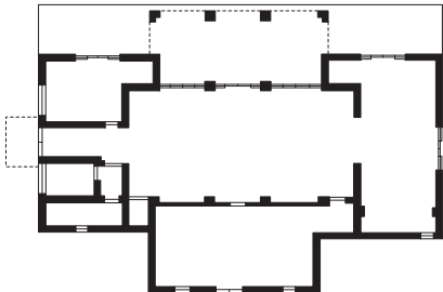
PLANTA ORIGINAL
