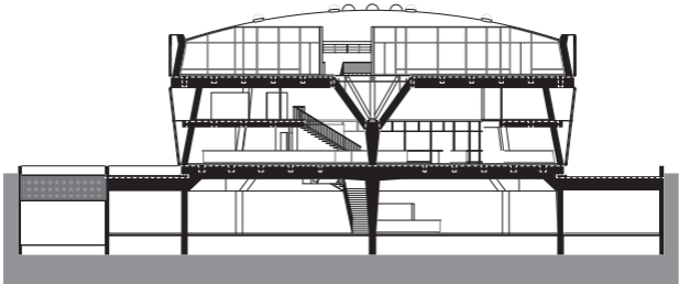
CORTE 0 5 10
