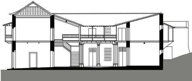
CORTE LONGITUDINAL
